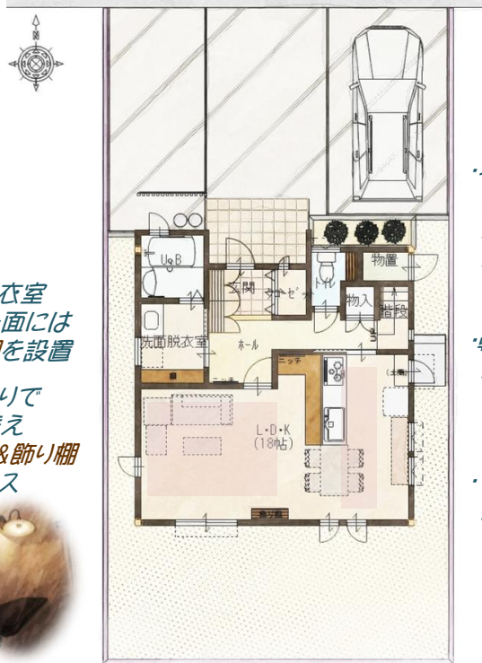
【1F配置兼平面図】
